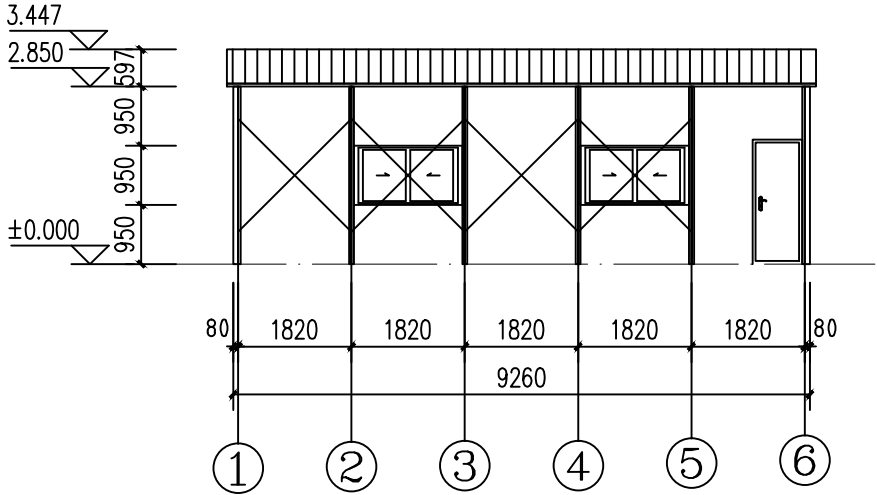
A-axis elevation
