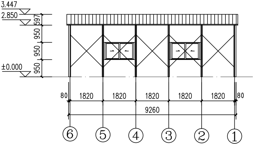
D-axis elevation
